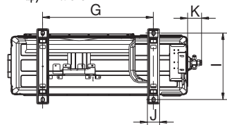
Наружный блок
